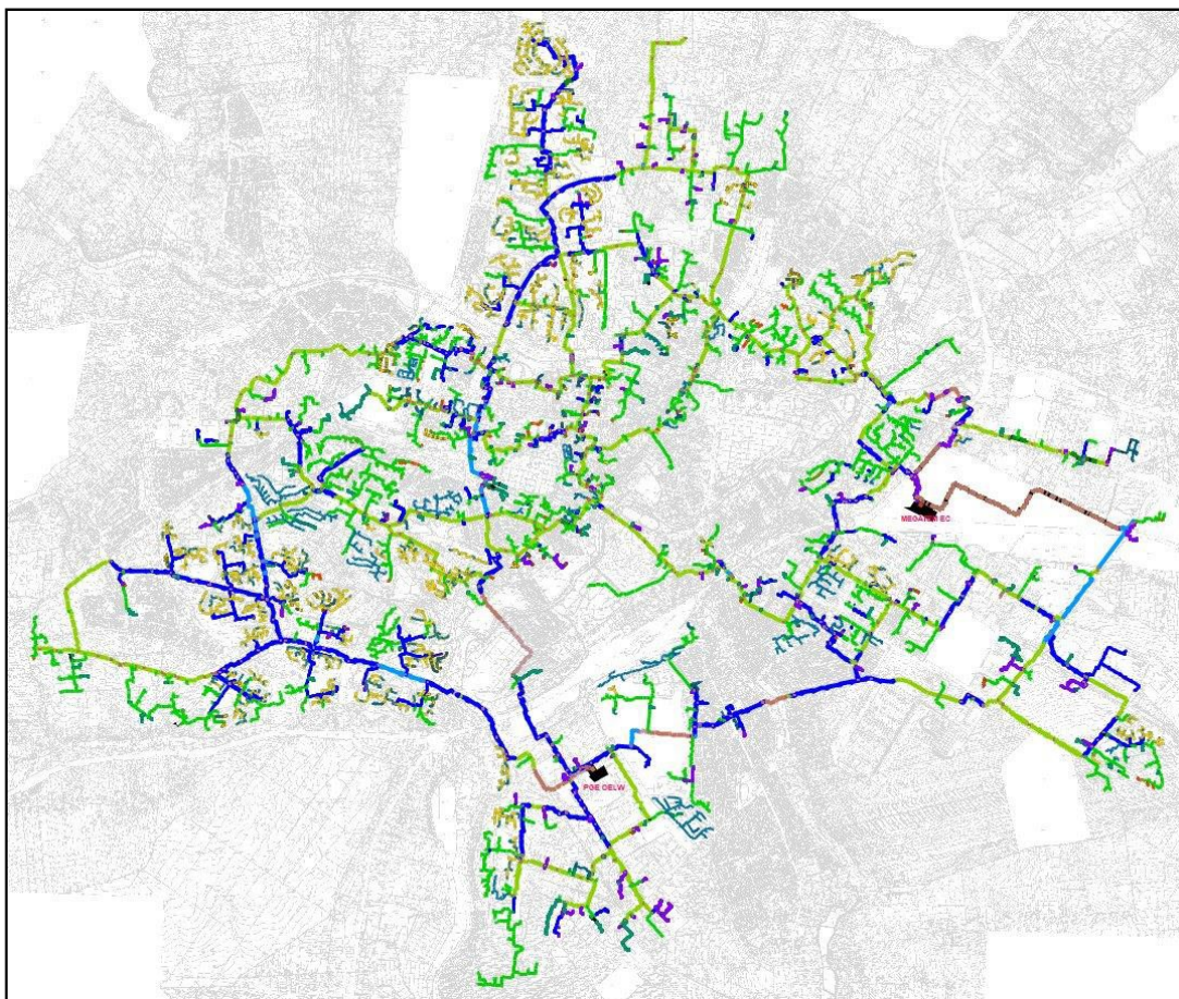
Ryc. 2 Schemat przebiegu miejskiej sieci ciepłowniczej w Lublinie
