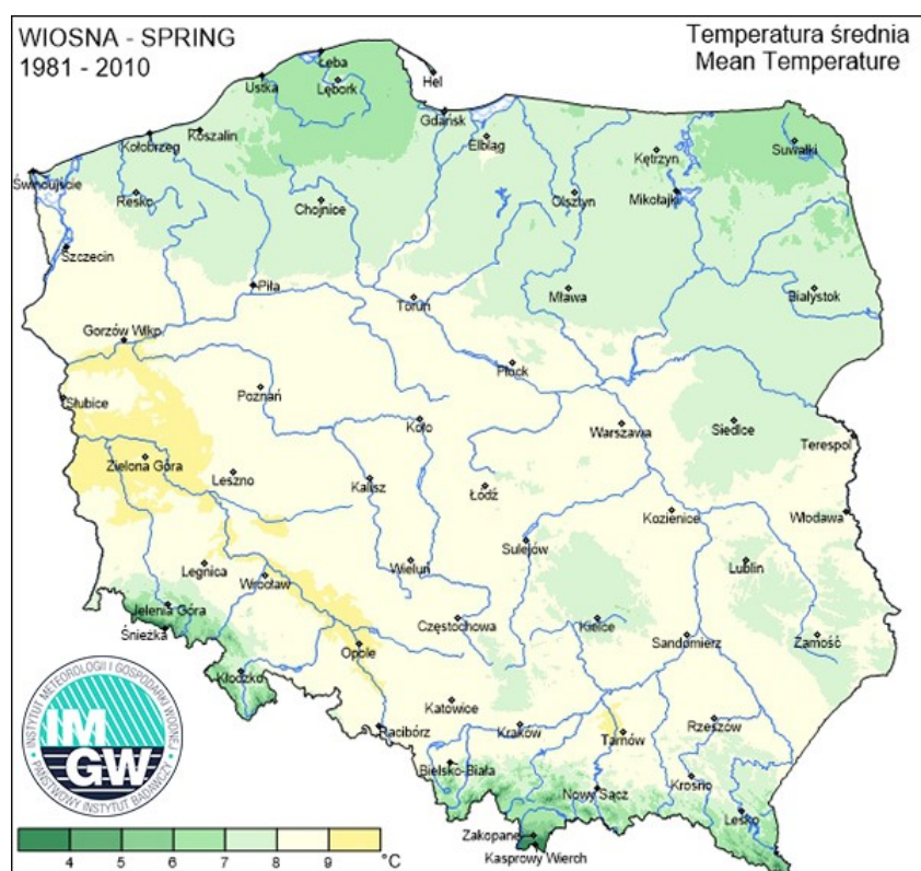
Ryc. 6 Rozkład średniej temperatury wiosną na terenie kraju (dane z wielolecia)
